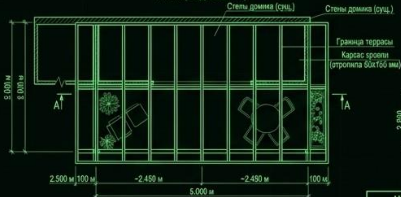
ПЛАН (ВИД С ВЕРХУ)
